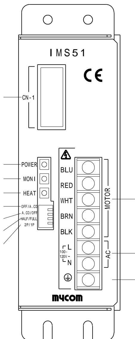
フロントパネル外形図
