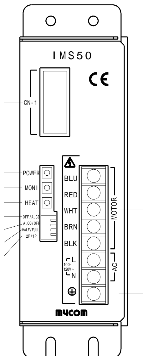
フロントパネル外形図
