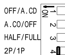
2パルス方式
