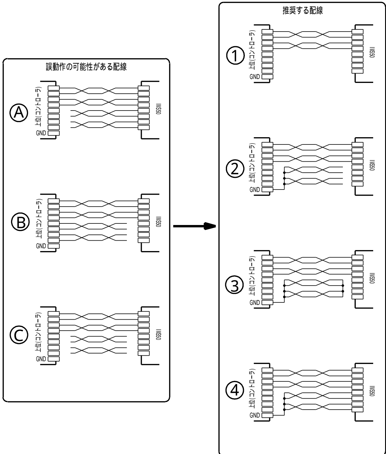
ツイストペア線配線図
